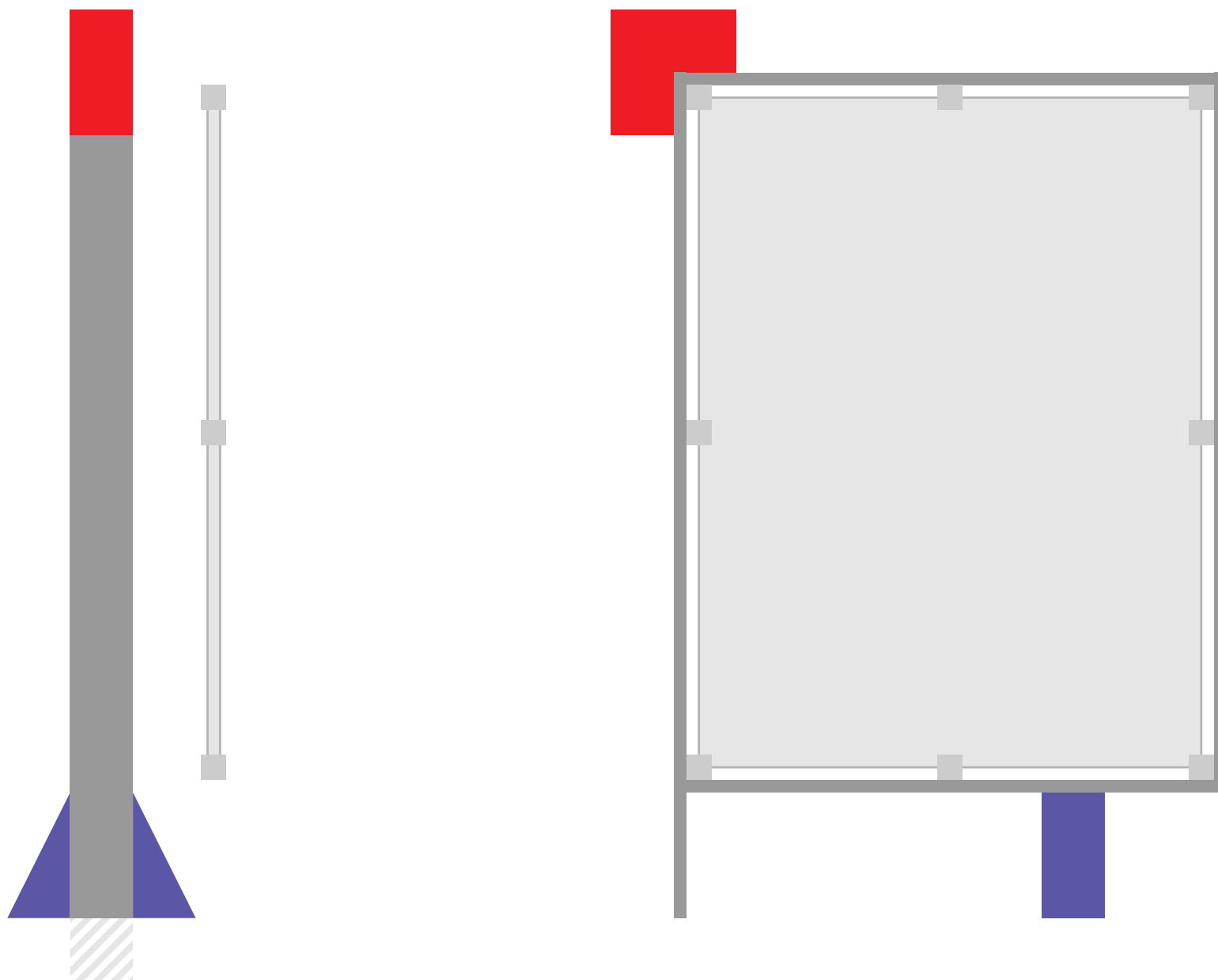
001 Mobilier extérieur d'affichage "à la française" (120 x 160 utile) – Profil et face
