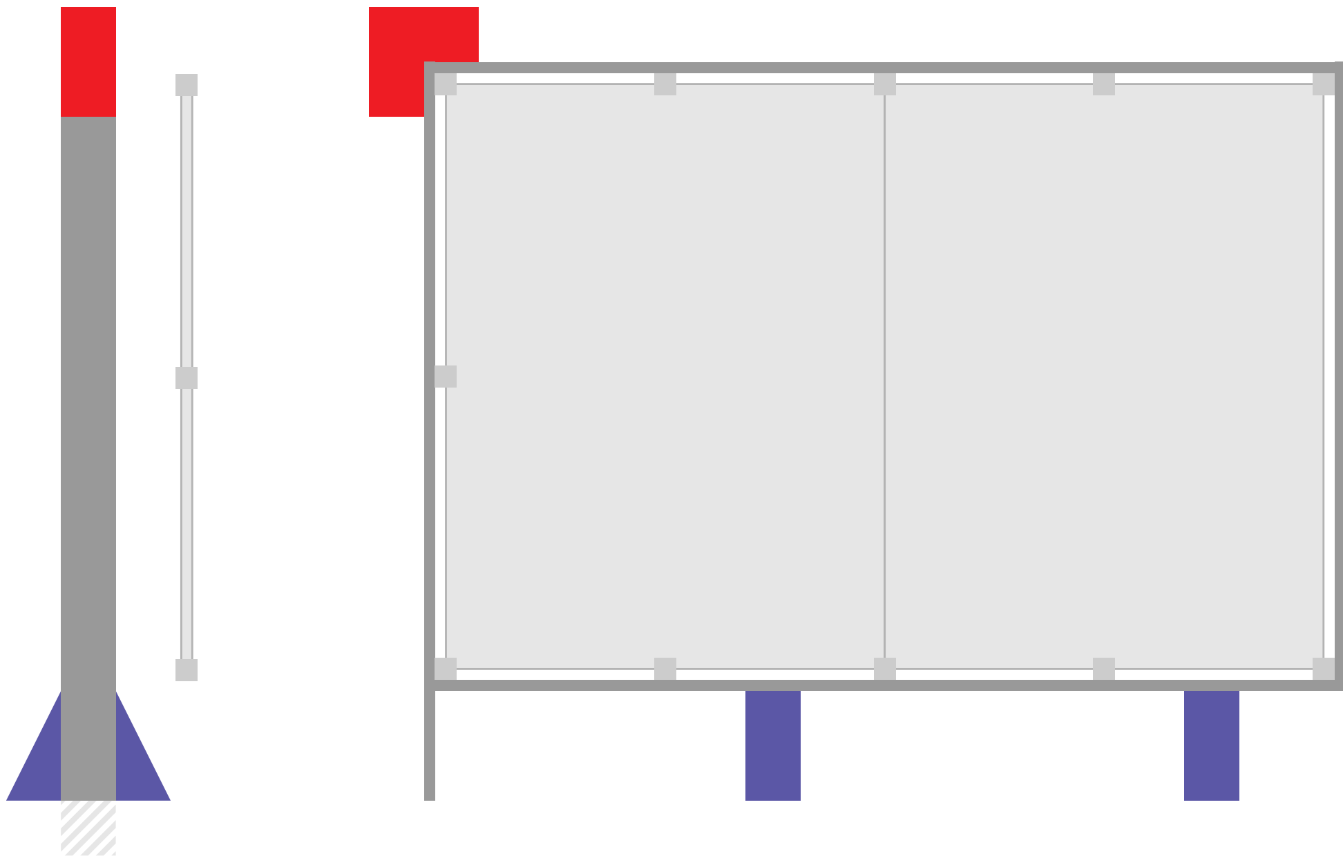
002 Mobilier extérieur d'affichage "à l'italienne" (240 x 160 utile) – Profil et face
